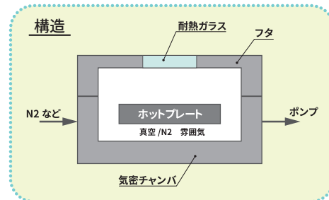
自動タイプ・半自動タイプ 真空ホットチャンバー
