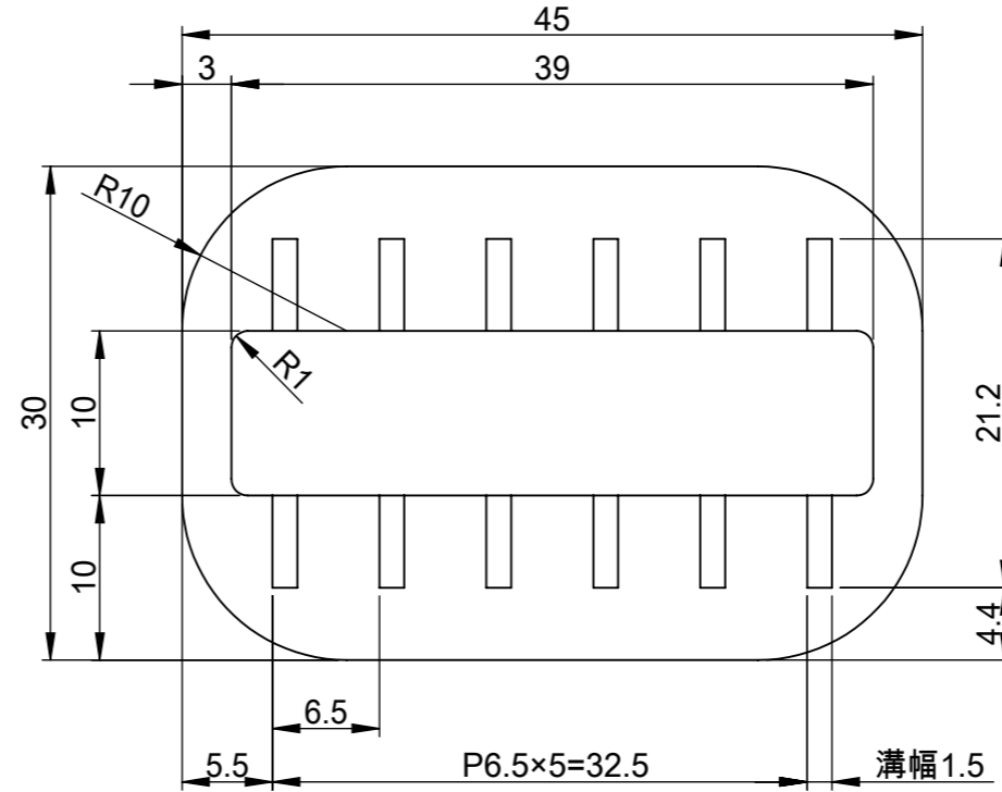
詳細図 B スケール 2 : 1
